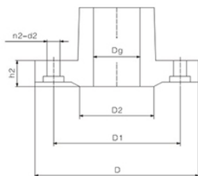
连接法兰
